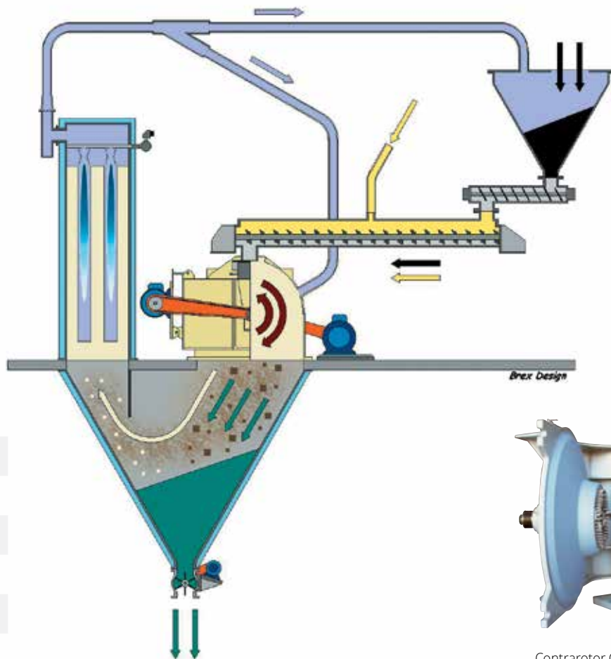
Contrarotor C30
